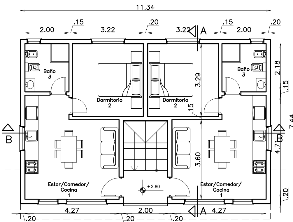
PLANTA ALTA
