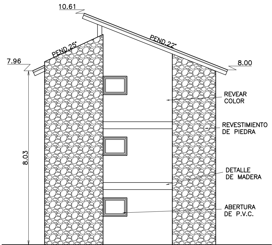
VISTA LATERAL DERECHA
