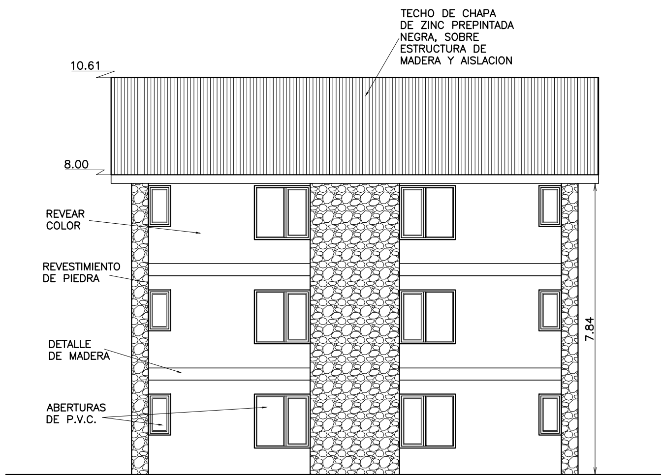
VISTA CONTRAFRENTE
