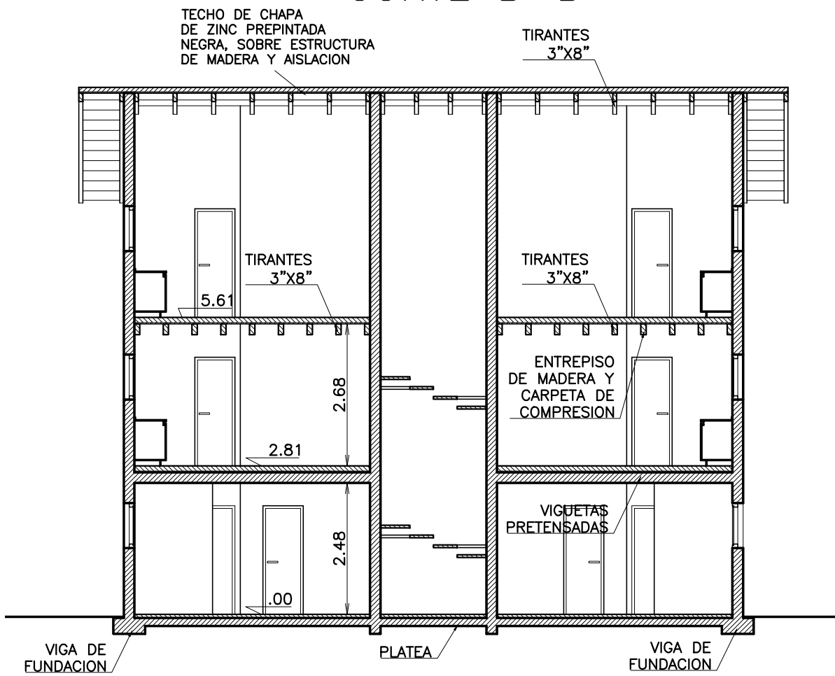
CORTE B-B
